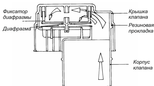
Клапан закрыт
