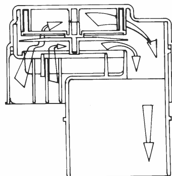
Клапан открыт
